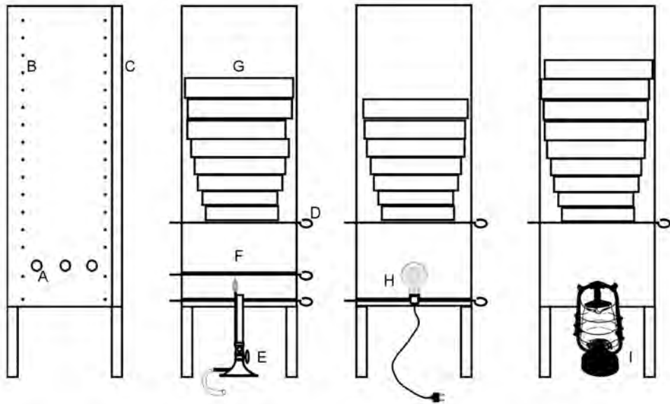
Fig. 41. Séchoir (vue latérale). A. Trous d'aération; B. Perforations pour les broches; C. Charnières. Dispositif au gaz (en coupe). D. Broches; E. Brûleur; F. Plaque de dissipation de chaleur; G. Tamis. Dispositif à l'électricité (en coupe). H. Soquet et ampoule 100 W. Dispositif au pétrole (en coupe). I. Lampe tempête.
